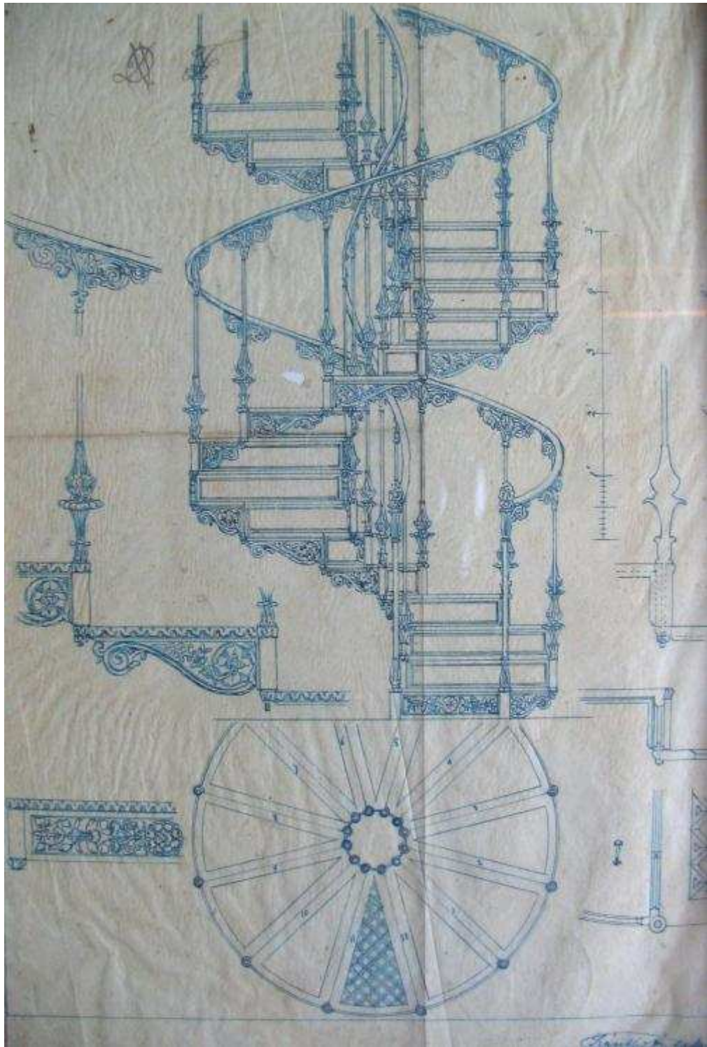
Csigalépcsőház terve
